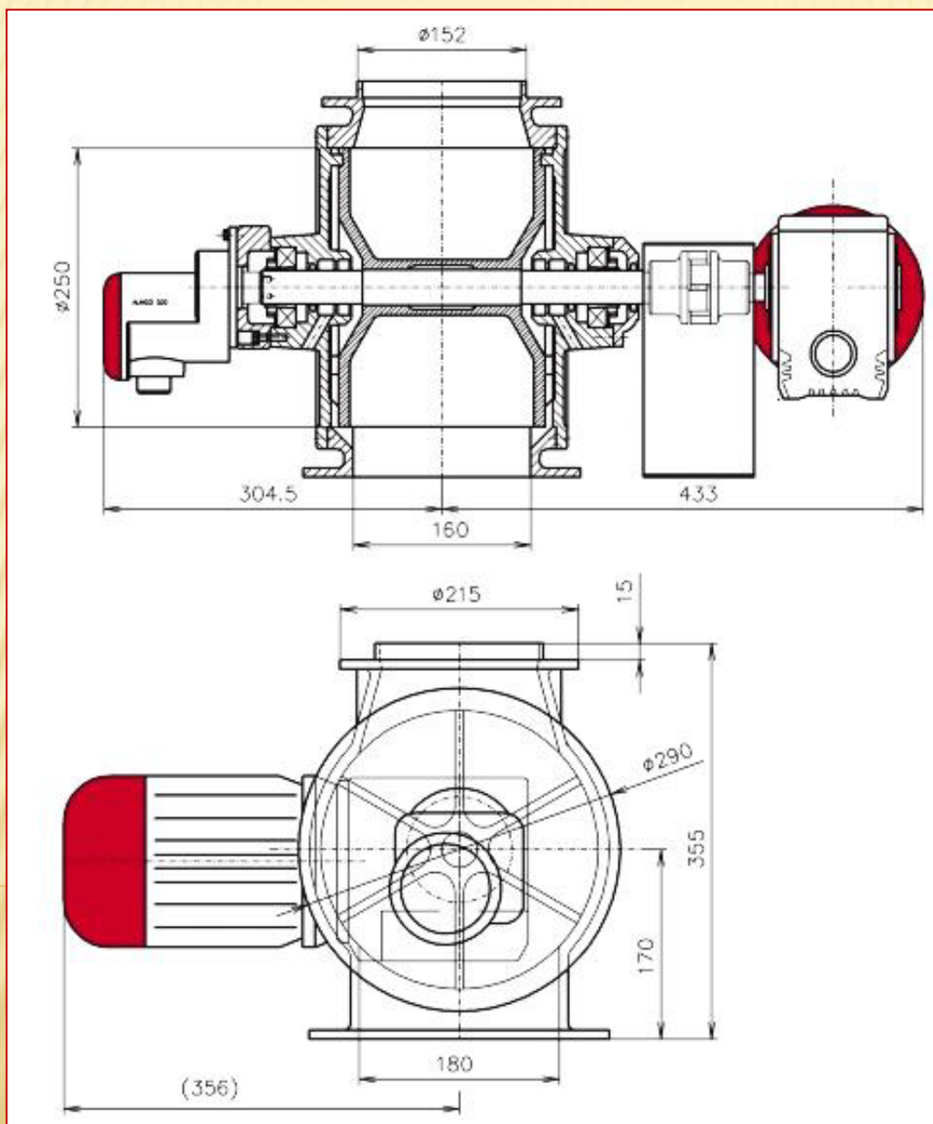
PT 250 s elektromotorem
